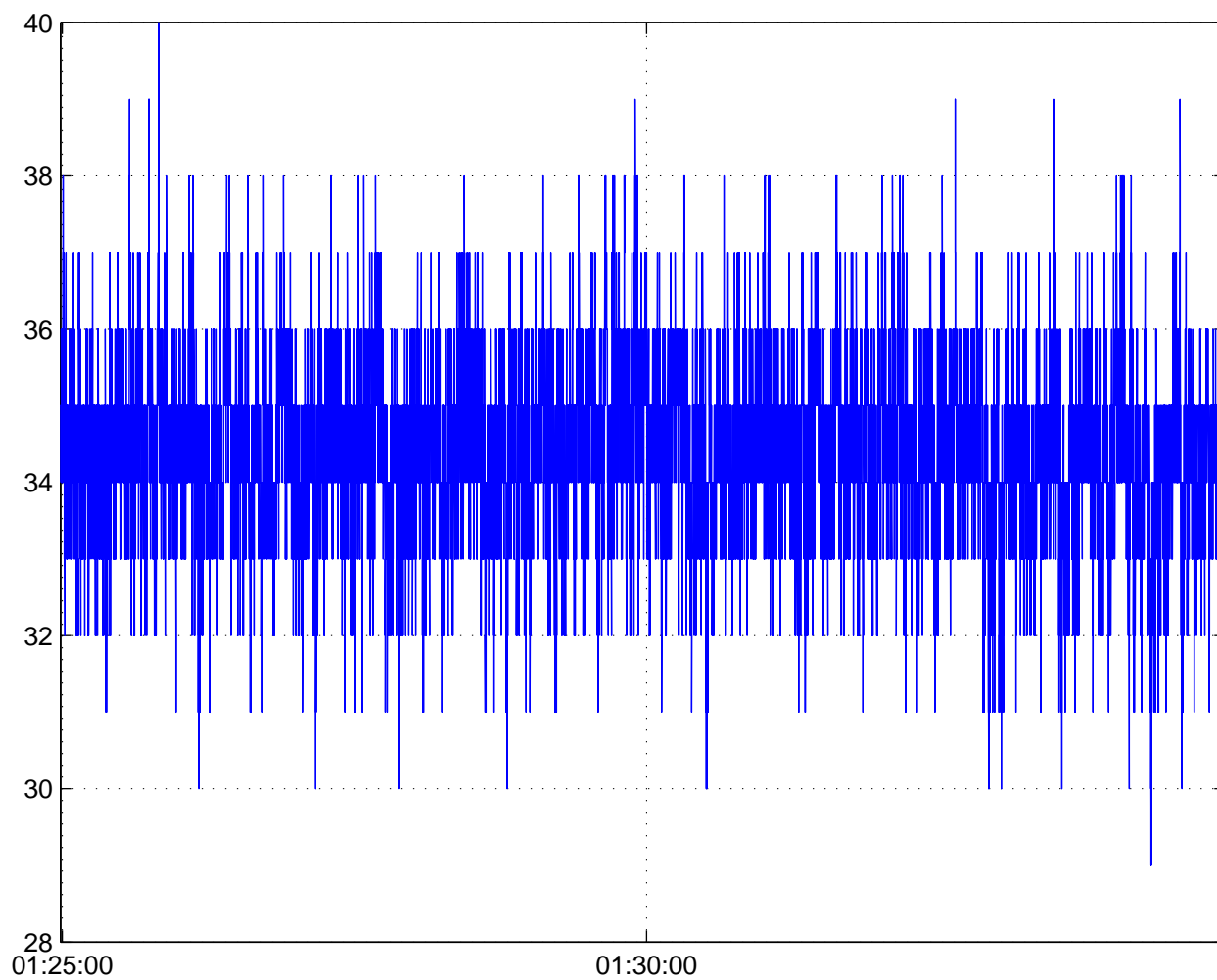
ATV tro FA, 2010-3-20 1:24:59 UT to 2010-3-20 1:34:57 UT
